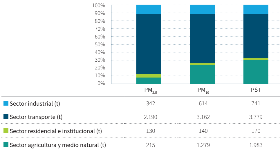
Gráfico 18. Contribución por sectores a las emisiones de partículas. Año 2010.
