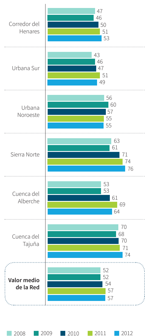
Gráfico 5. Comparativa por zonas de la media anual de ozono. Periodo 2008-2012 ( \mu\text{g}/\text{m}^3 )
