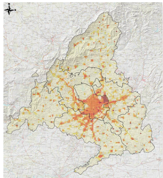
Imagen 3. Inventario de emisiones de CO. Año 2010.
