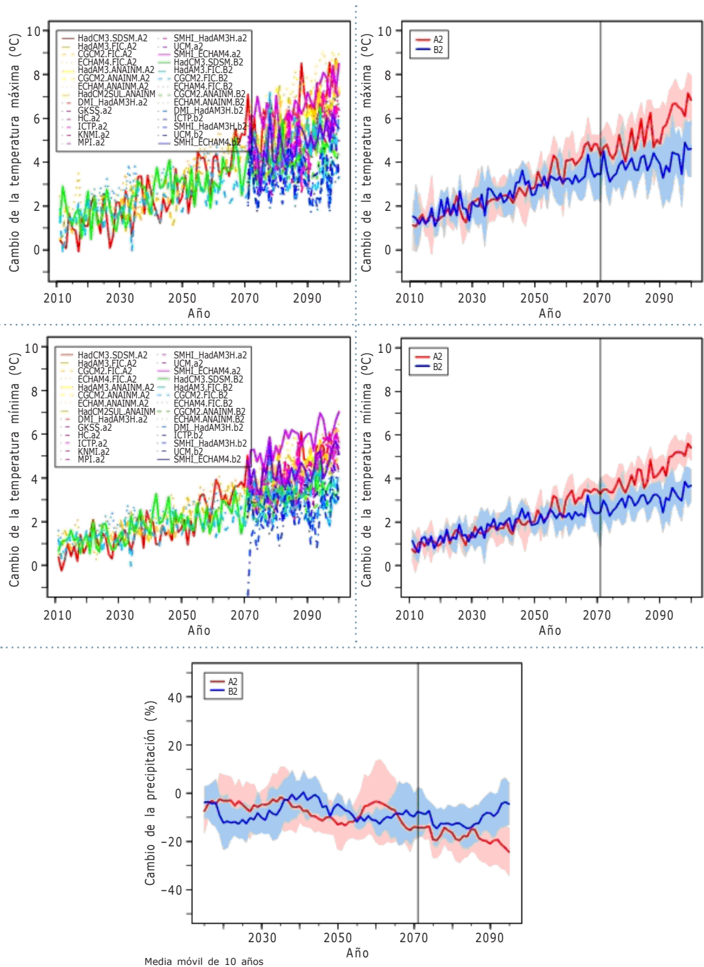
Gráfico 43. Definición de las desviaciones de temperatura media anual de las máximas (°C), temperatura media anual de las mínimas (°C) y precipitación anual media (%) de los escenarios regionalizados para la Comunidad de Madrid.
